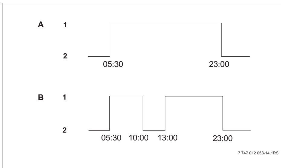
fig. 16 Introdução de pontos de comutação para interromper uma fase de aquecimento
