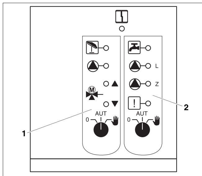
fig. 22 Módulo de função FM441
