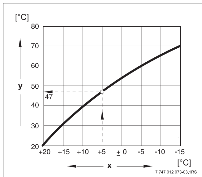
fig. 3 Curva característica de um circuito de aquecimento (exemplo)
