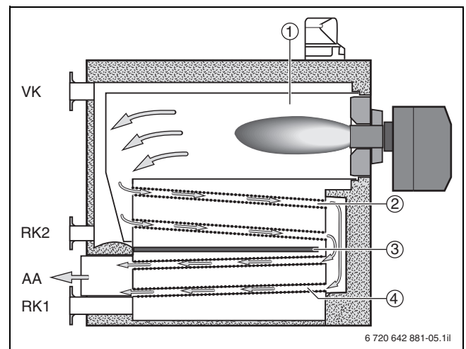
fig. 1 Esquema de funções do curso de gás de aquecimento em caldeiras de condensação Logano plus SB325
