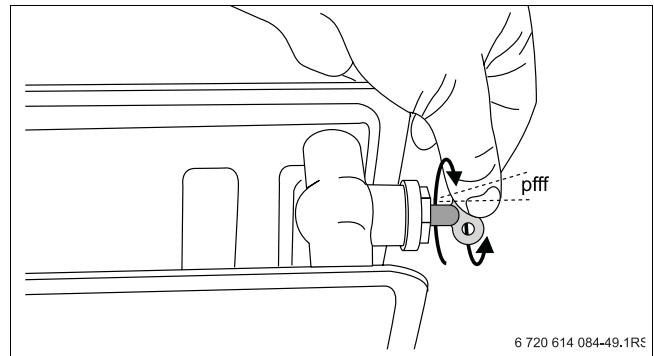
Fig. 14 Purgar os radiadores
