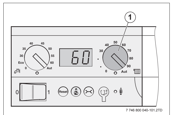
Fig. 7 Painel de comando do controlador básico
