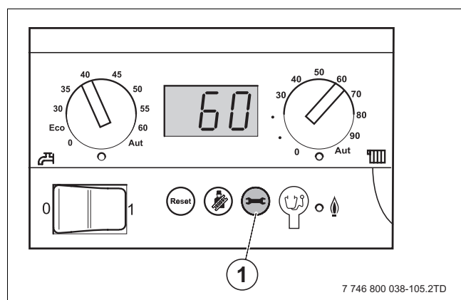
Fig. 16 Painel de controlo do controlador básico
