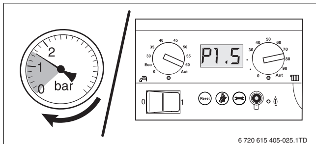
Fig. 10 Indicação de pressão analógica/digital
