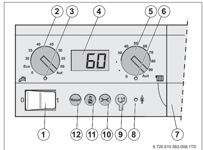
Fig. 5 Painel de controlo – Elementos de comando
