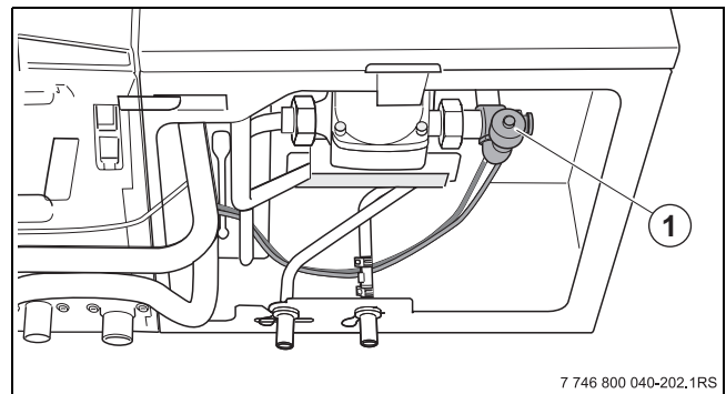
Fig. 15 Drenar acumulador de micro-acumulação
