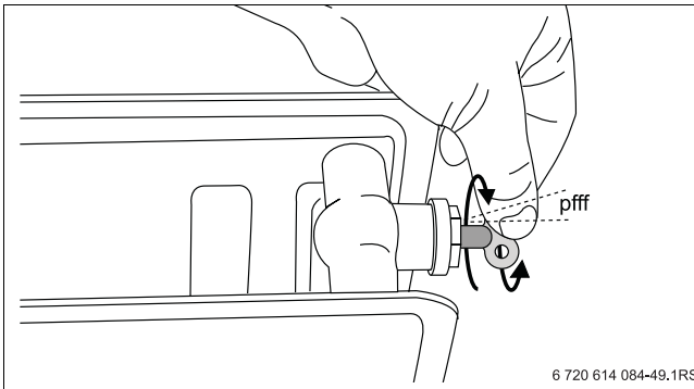
Fig. 12 Purgar os radiadores.
