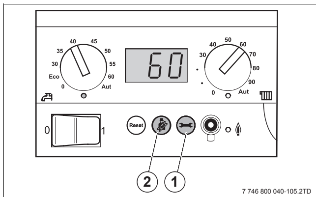
Fig. 8 Painel de controlo do controlador básico
