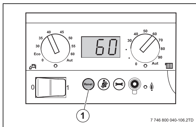
Fig. 17 Controlador básico BC10
