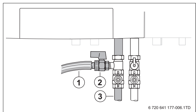
Fig. 11 Abrir a torneira de enchimento e drenagem
